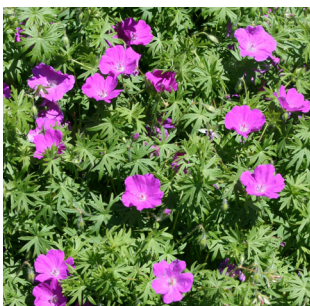
Geranium sanguineum
